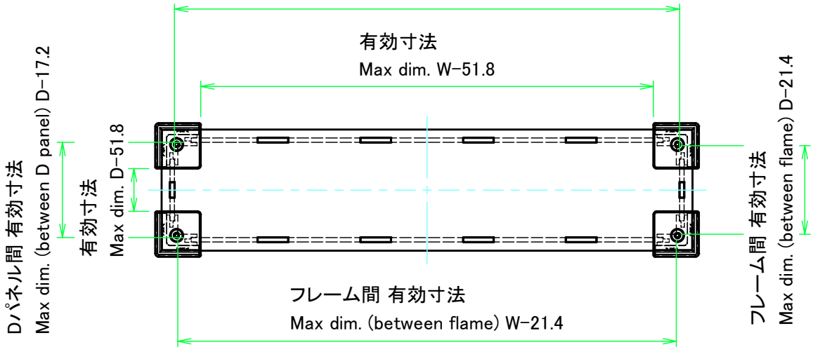
Wパネル間 有効寸法 Max dim. (between W panel) W-17.2
